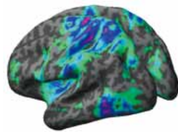
〔運動中のヒトの脳活動〕 動き回るターゲットを目で見て、手を動かして追跡しているときの脳活動(脳を左後方から見た図)
